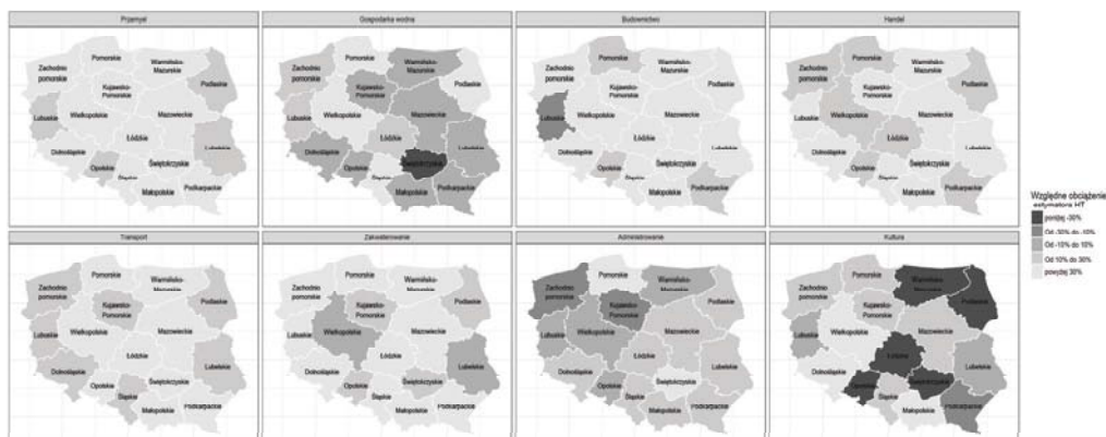
Estymator Horvitz-Thompsona
